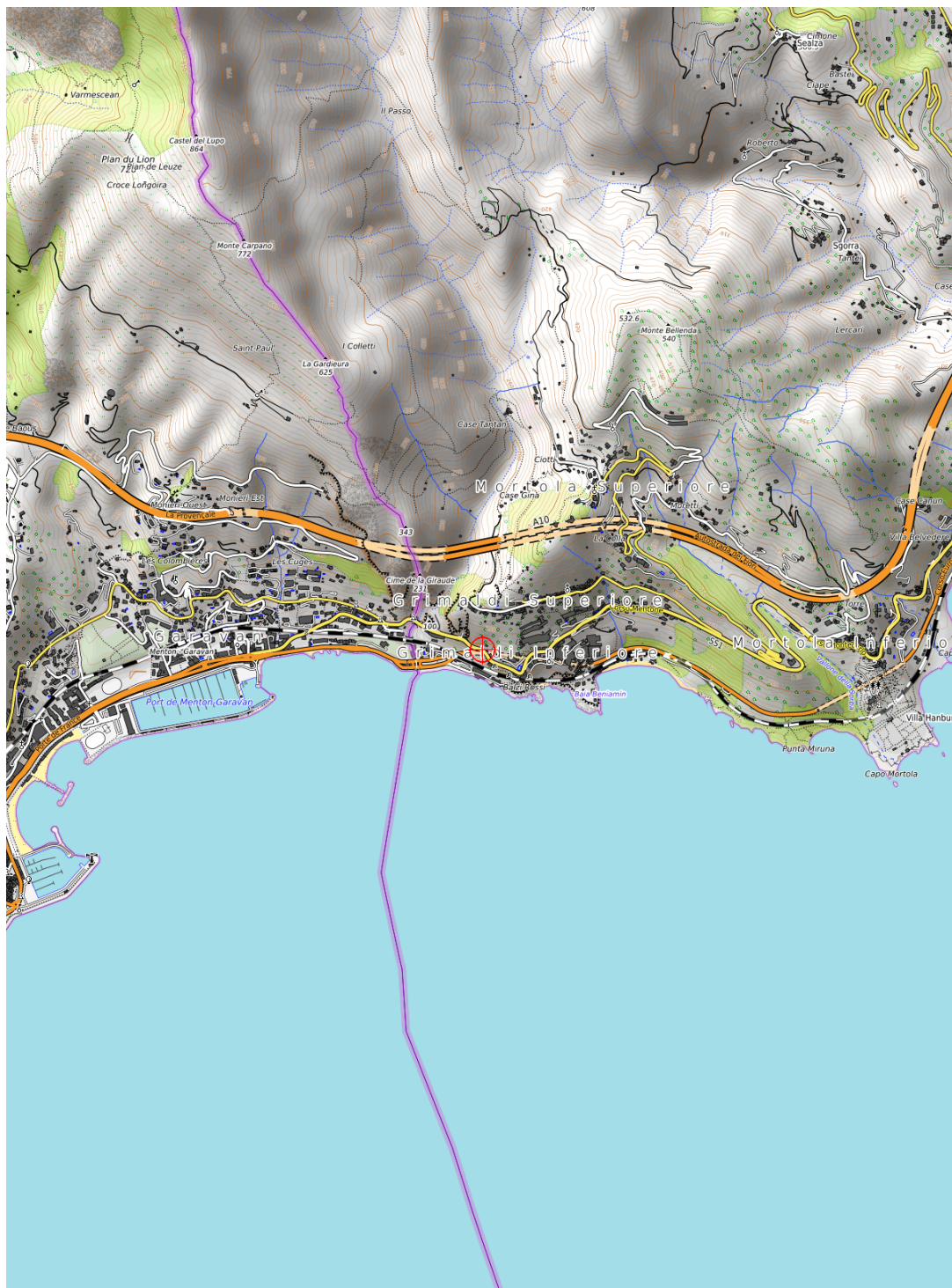
LIL1189 estratta da www.catastogrotte.net giovedì 11 giugno 2026 - 06:00
